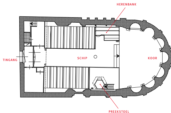
PLATTEGROND KERK THESINGE
