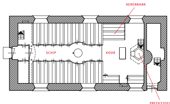
PLATTEGROND SINT GEORGIUSKERK STITSWERD
