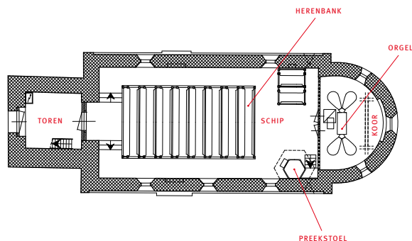
PLATTEGROND KERK MARSUM
