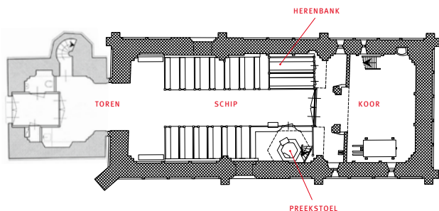
PLATTEGROND MARIAKERK KREWERD
