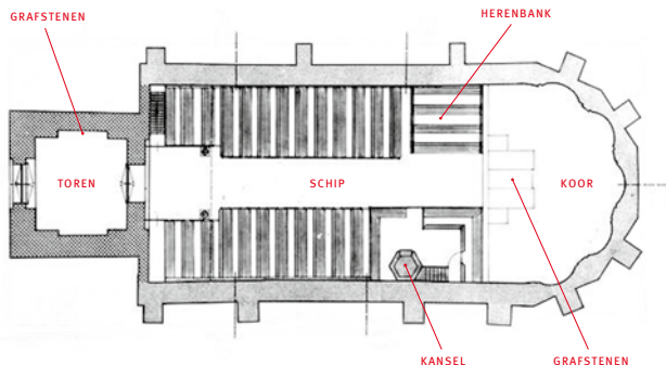
PLATTEGROND NEDERLANDS HERVORMDE KERK GARNWERD
